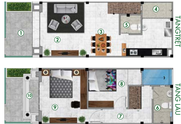
MẪU NHÀ KR ĐIỂN HÌNH (DT: 48m 2 )
